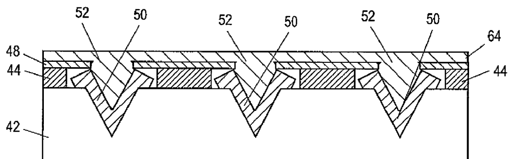
FIG. 5I
