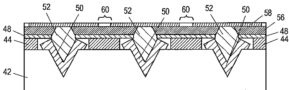
FIG. 5F
