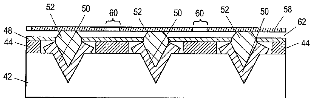
FIG. 5G
