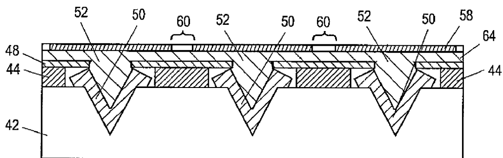
FIG. 5H
