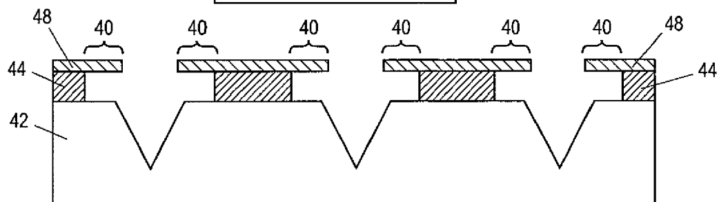
FIG. 4D
